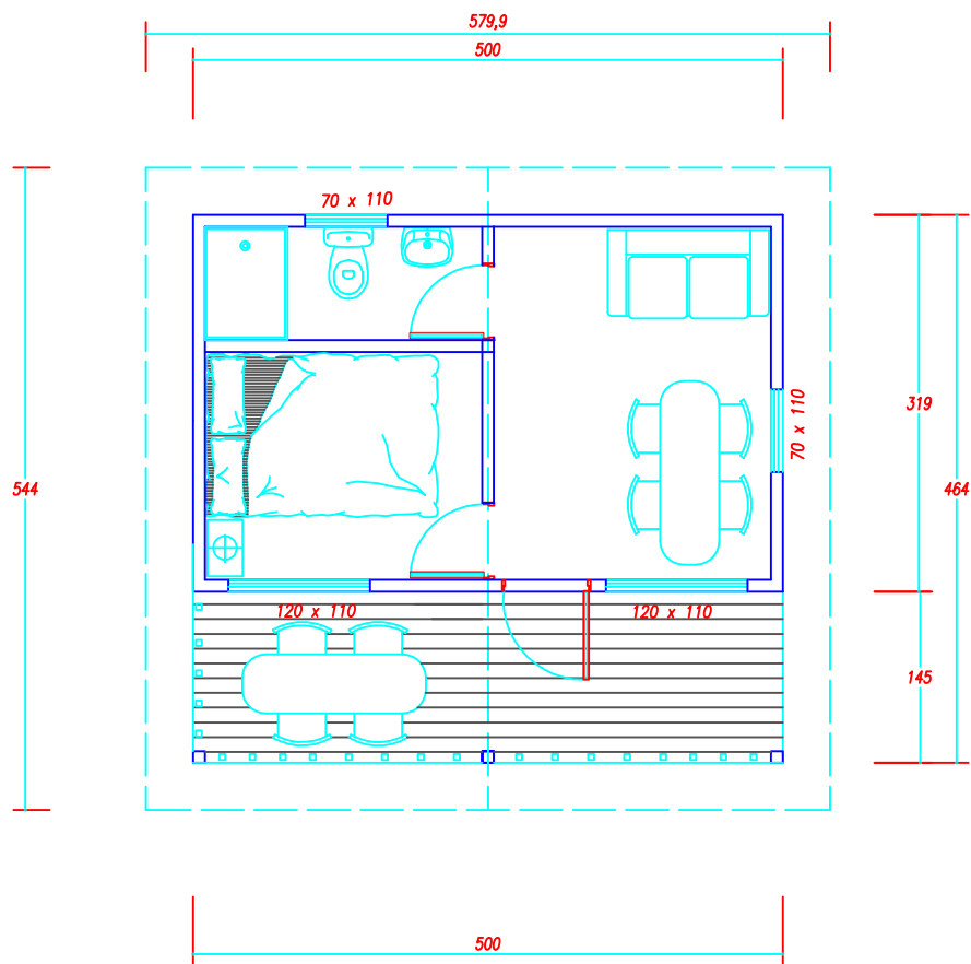
PLANTA DE ARQUITECTURA
