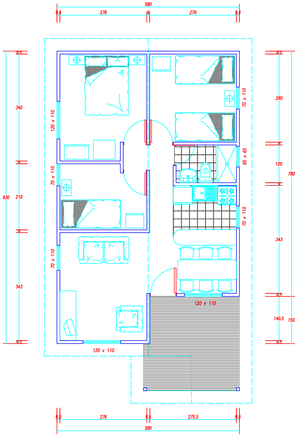
PLANTA DE ARQUITECTURA
