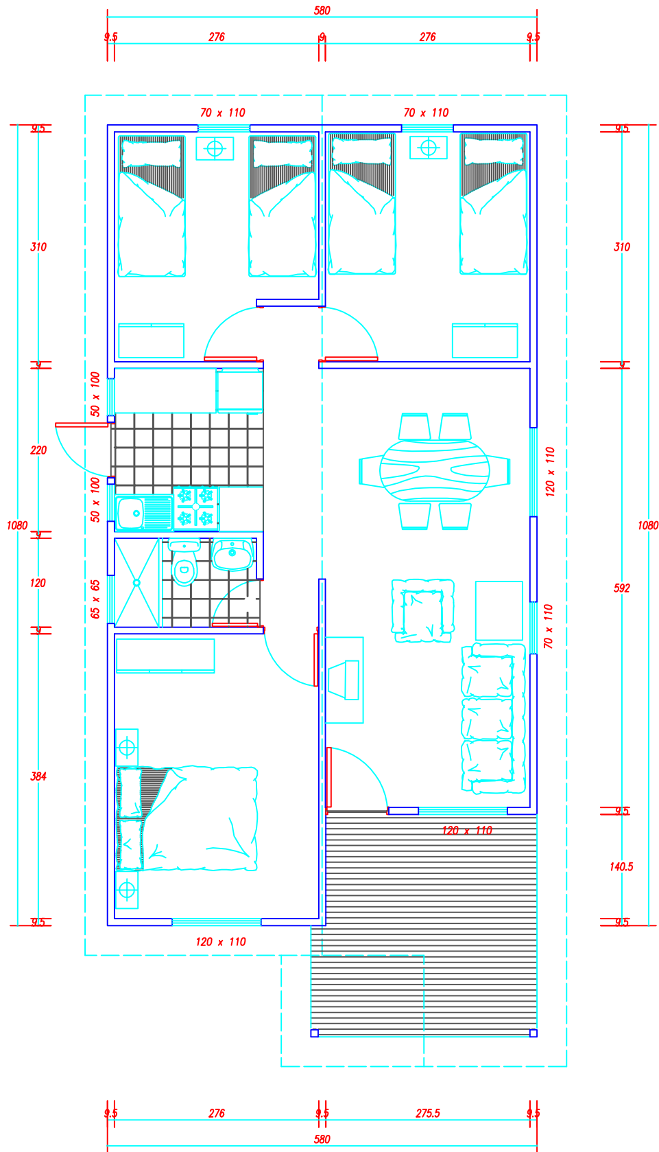
PLANTA DE ARQUITECTURA
