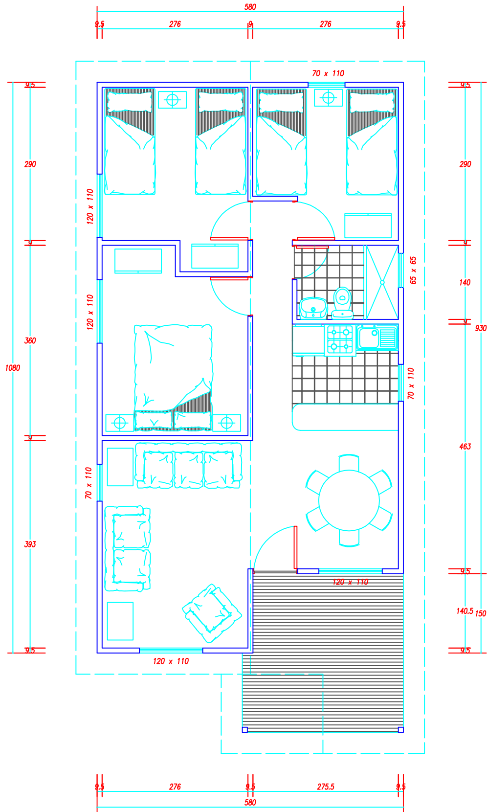
PLANTA DE ARQUITECTURA
